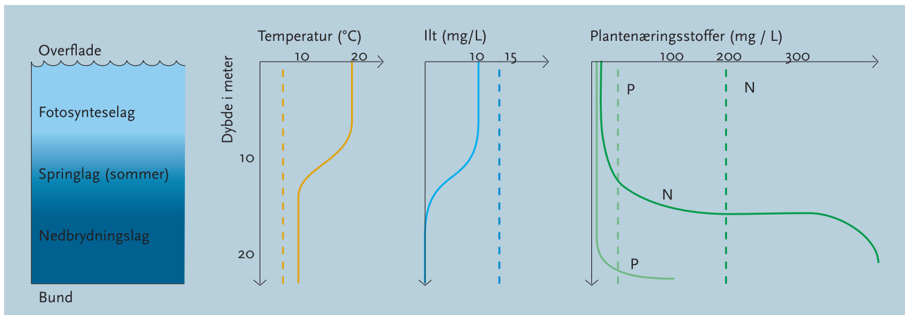
Figur 187. Temperatur, iltindhold og næringsstofindhold i en dyb sø.
