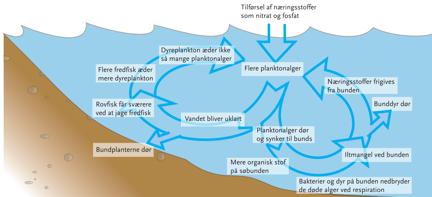
Figur 190. Onde cirkler i søer.
