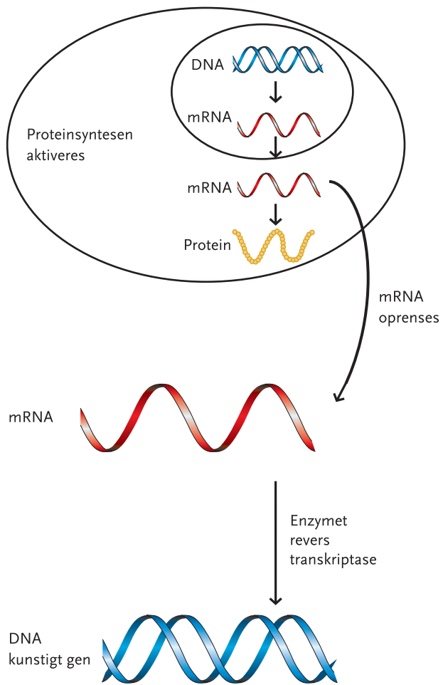
Figur 216. Copy-DNA-metoden.
