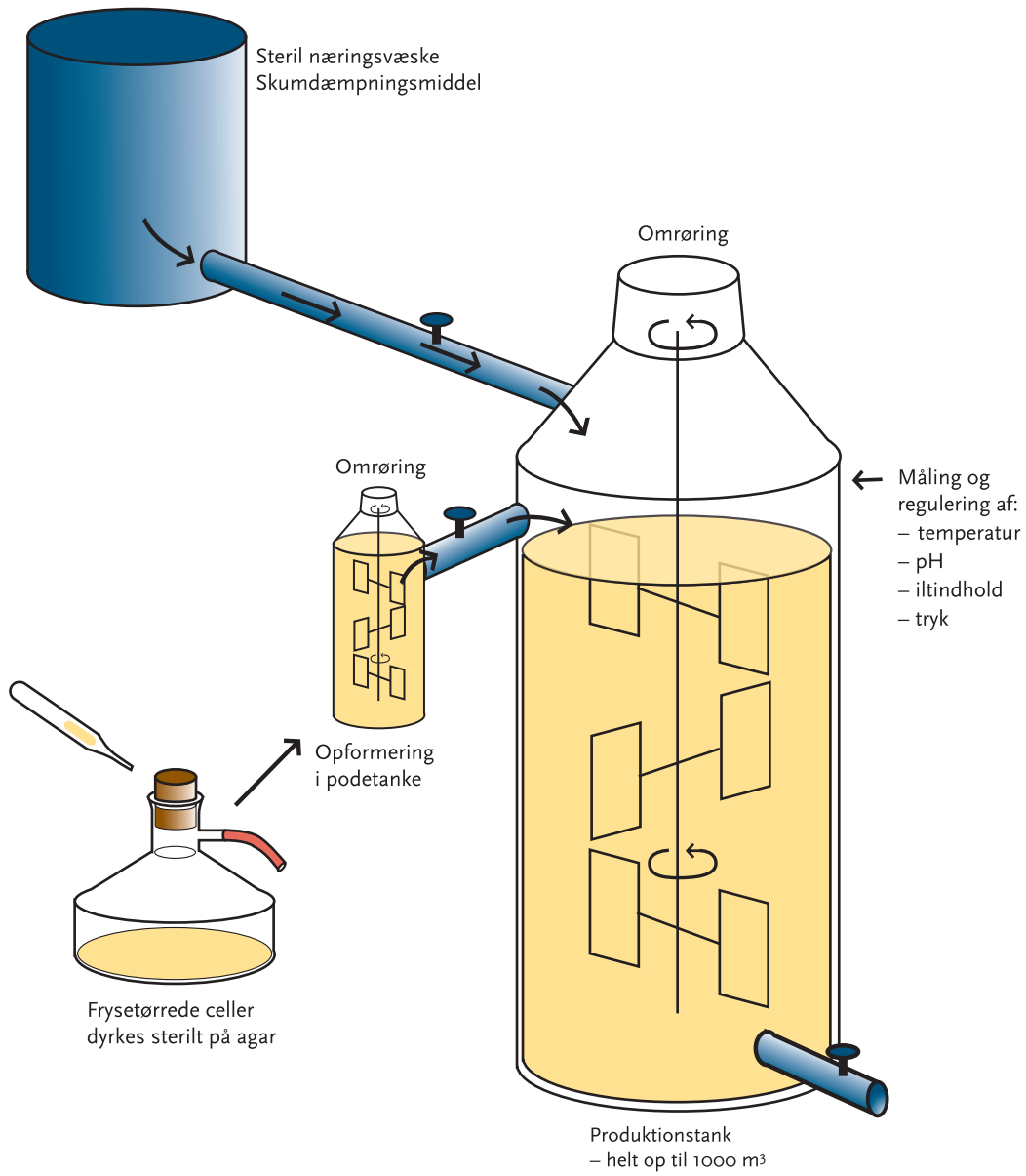
Figur 219. Oversigt over gæringsprocessen.
