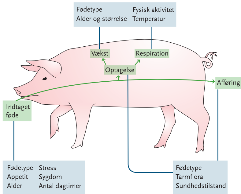
Figur 232. Faktorer som påvirker udnyttelsen af foder i svin.
