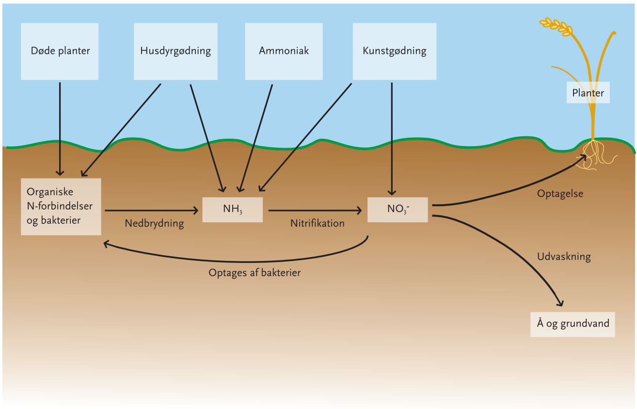
Figur 233. Nitrogenholdige stoffers omsætning i jorden.
