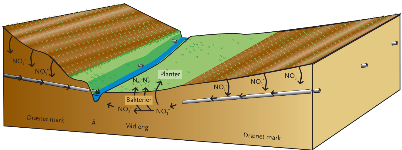
Figur 237. Nitratfjernelse i en våd eng.
