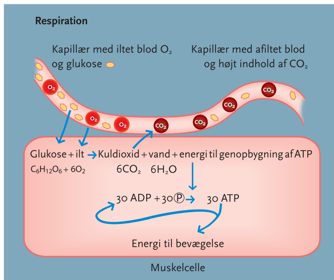
Figur 52. Respirationsprocessen.
