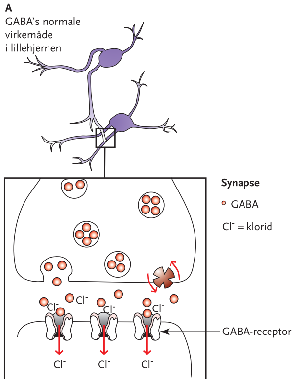
Figur 89. Alkohol øger indstrømningen af \text{Cl}^- og dermed afslapper nerven.
